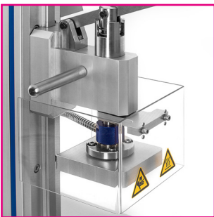
Siegelstempel-Heizblock
