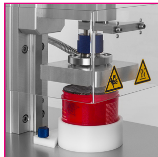
Tiegelaufnahme (z.B. für Kosmetiktiegel)
